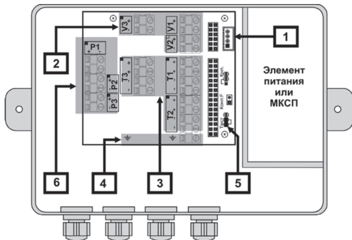
Рисунок Б.1 Внешний вид монтажного отсека KAPAT-306-1
