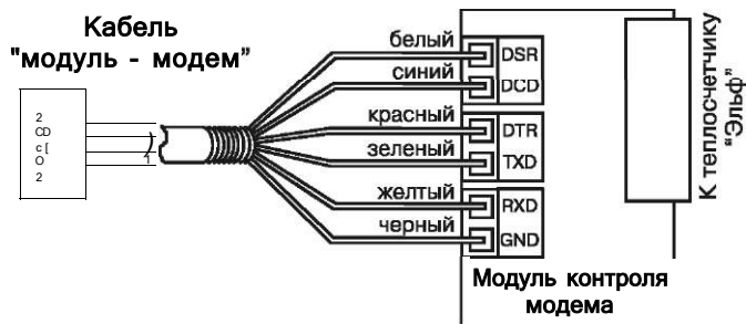
Рисунок 1 Схема подключения модуля к модему
