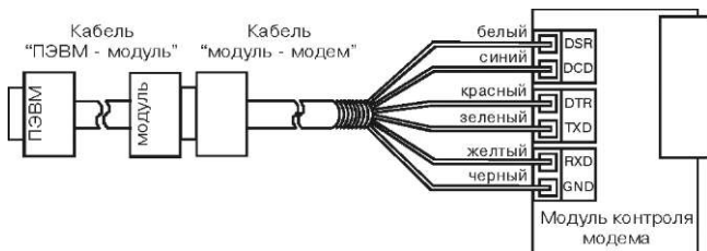
Рисунок 5 Схема подключения модуля контроллера модема к компьютеру
