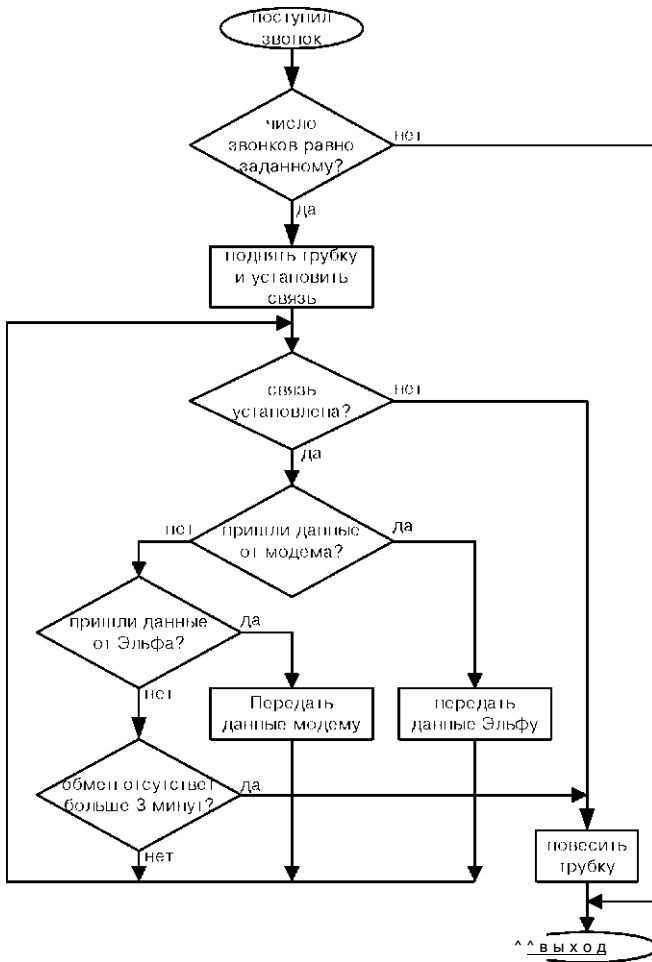
Рисунок 3 Блок-схема алгоритма обработки звонка
